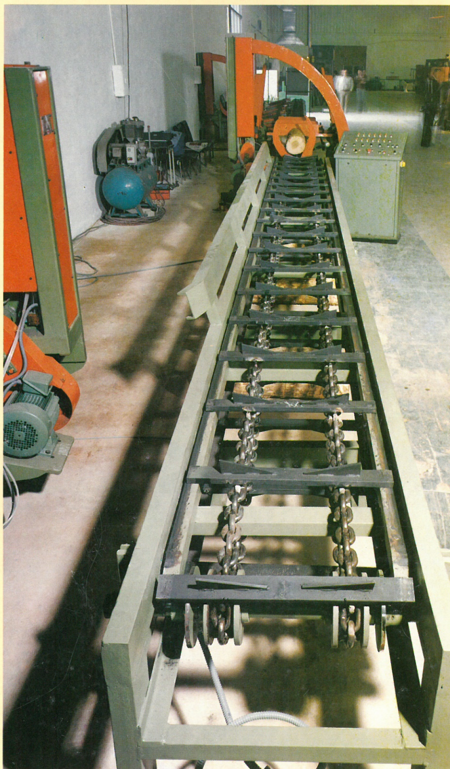
TRONZADORA L.M. 1.100 MARCA LABRADOR. Detalle doble arrastre por cadenas y pupitre de mandos.
